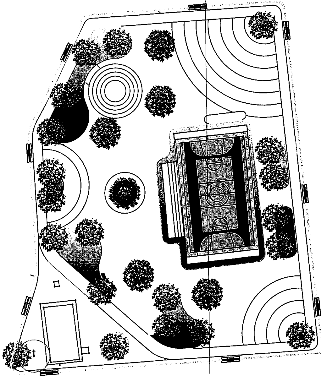
PLANTA URBANÍSTICA - PRAÇA SANTO ANTÔNIO Escala: 1:200
