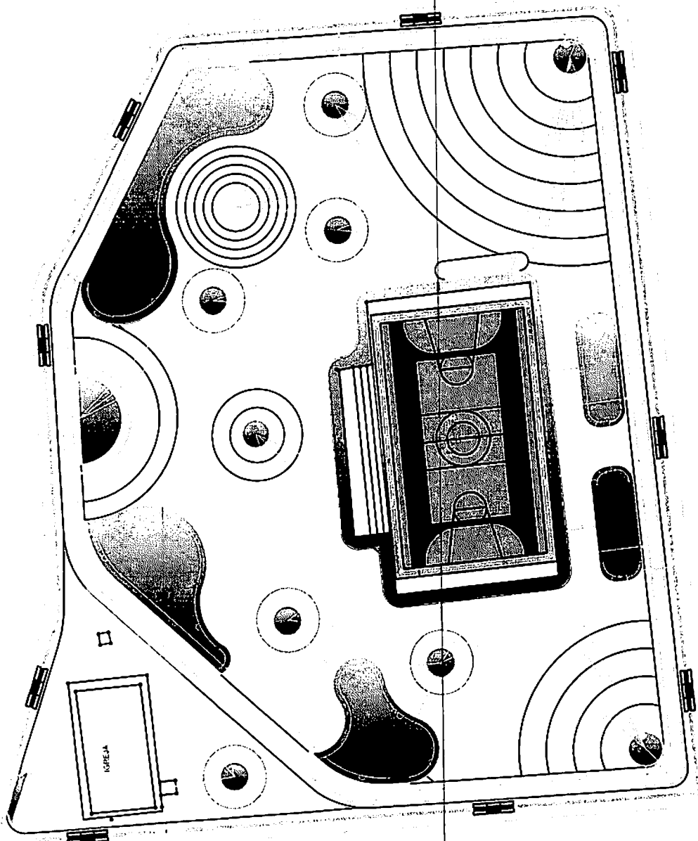
○ PLANTA DE GEOMÉTRICA - PRAÇA SANTO ANTONIO ESC.: 1/200
